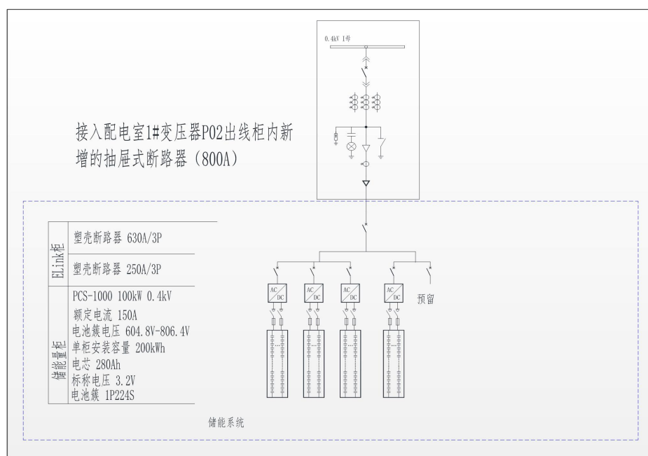
储能接入拓扑图（示范图例）
