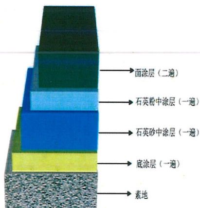
(四) 产品结构图:
